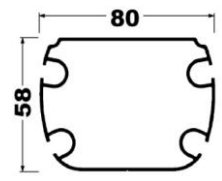
profil αντιβάρου bottom bar profile
