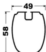
κόντρα / middle bar
