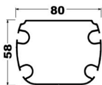
αντίβαρο / bottom bar
