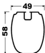
κόντρα / middle bar
