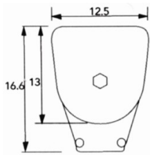
στήριξη σε οροφή roof fixing
