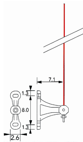
βάση στήριξης συρματόσχοινου wire rope support
