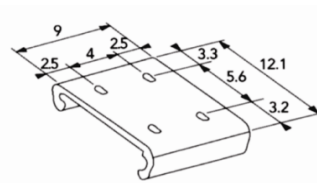
βάση στήριξης τοίχου - οροφής wall - roof support
