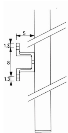
βάση στήριξης οδηγού side guide support
