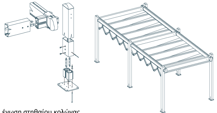
ένωση στηθαίου κολώνας beam & column joint
