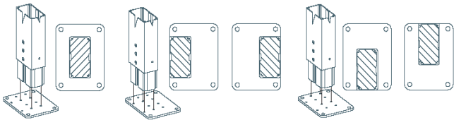
βάση στήριξης κολώνας column ground support
